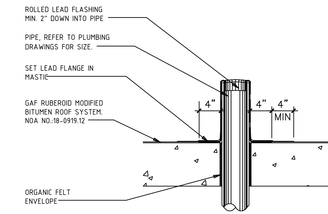
① PIPE PENETRATION DETAIL SCALE: N.T.S.
