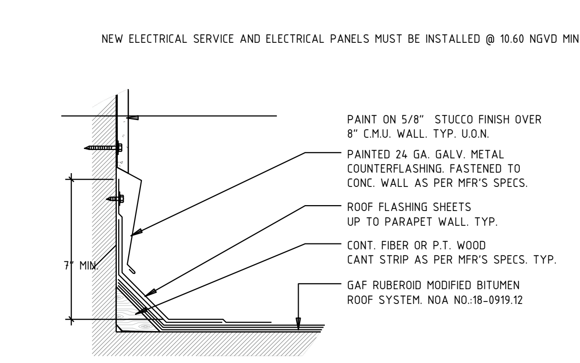
③ FLASHING DETAIL SCALE: N.T.S.
