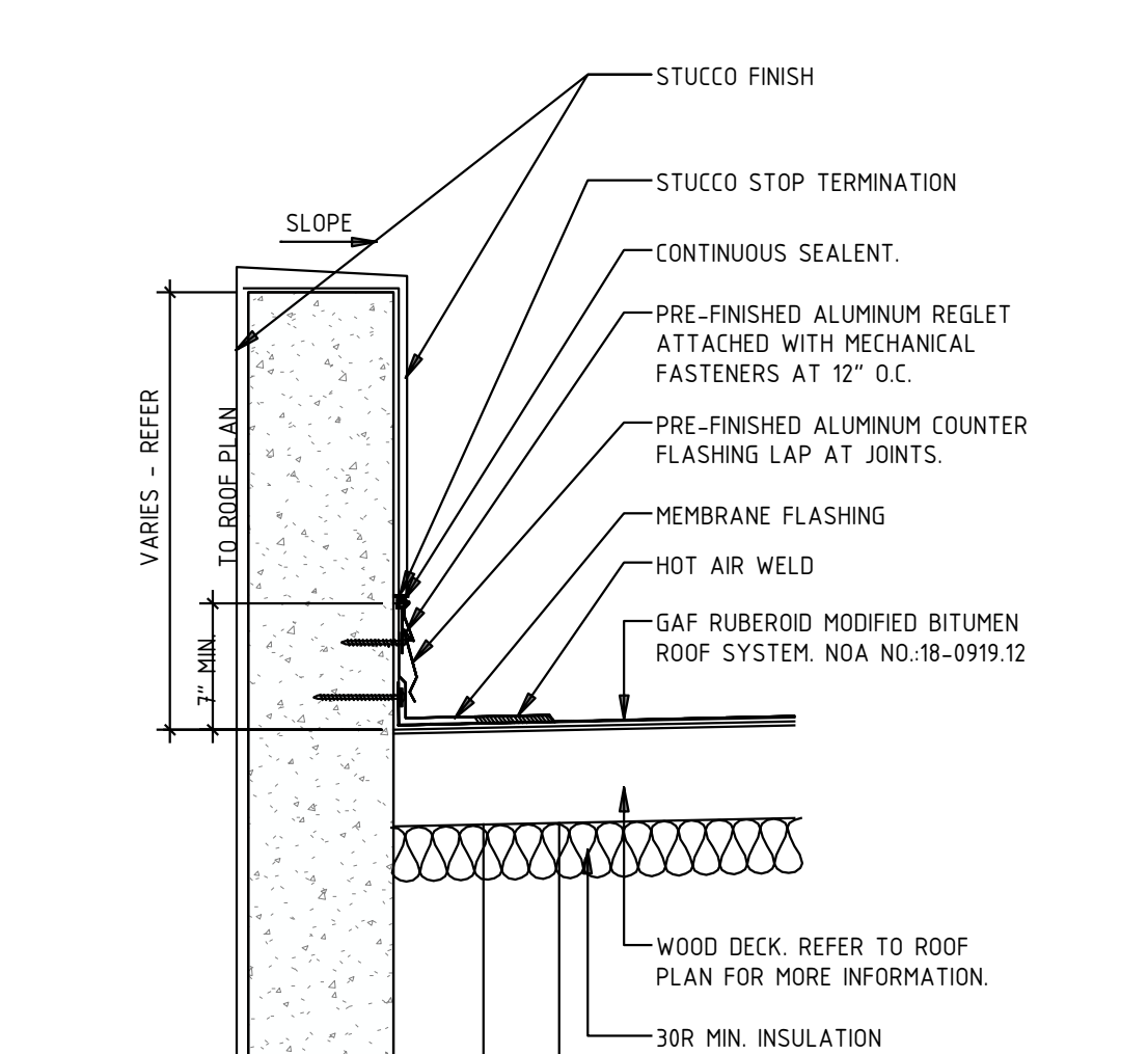
⑨ ROOF PARAPET DETAIL SCALE: N.T.S.
